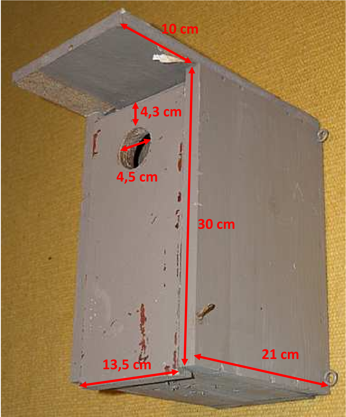
Målene til vendehalskassa:
